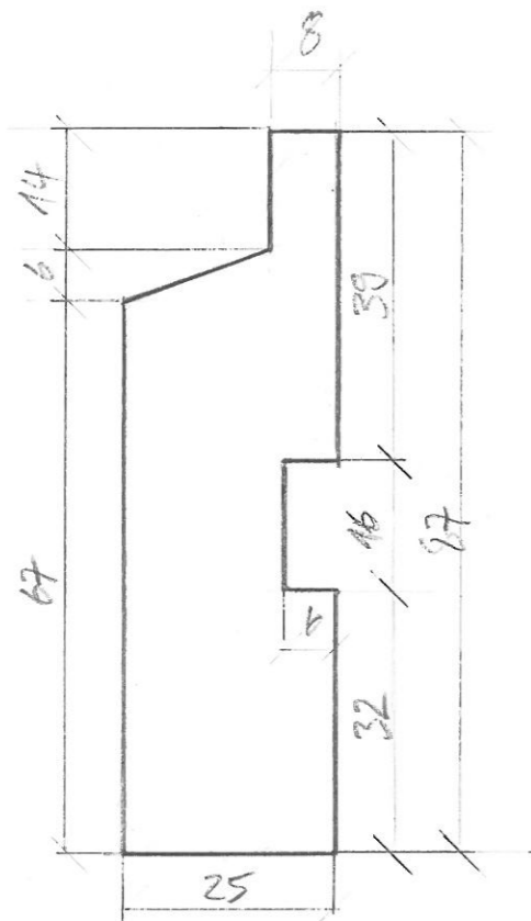
Detailansicht Seitenkeil, Länge 318
