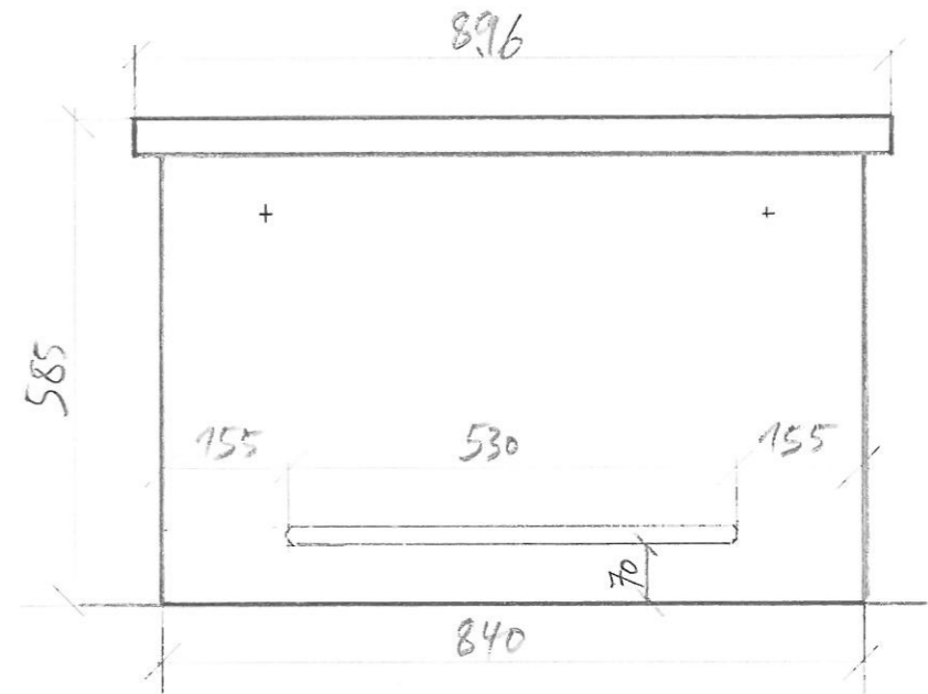
Vorderansicht, beide Seiten gleich
